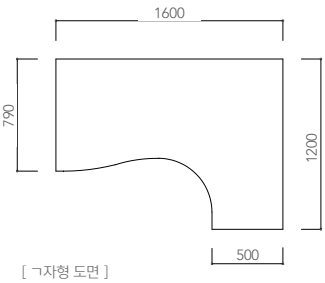
[ ㄱ자형 도면 ]
